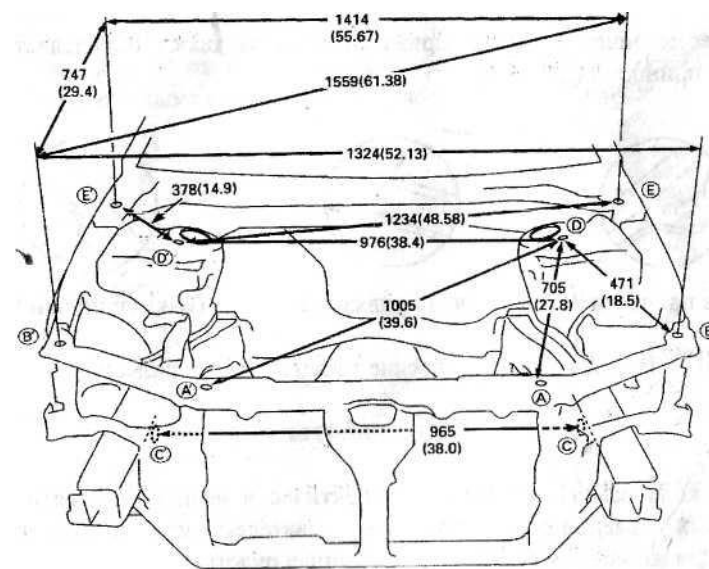
Рис. 2.2. Размеры передней части кузова
