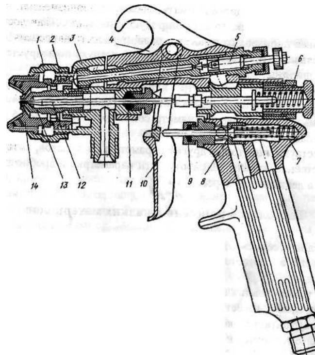
Рис. 7.1. Устройство окрасочного пистолета (краскопульт): 1 - распылительная камера; 2 - гайка накидная; 3 - корпус распылительной головки; 4 - корпус краскопульты; 5 - регулятор раскрытия факела; 6 - пружина иглы; 7 - пружина воздушного клапана; 8 - воздушный клапан; 9 - уплотнение воздушного клапана; 10 - курок; 11 - уплотнение иглы; 12 - игла; 13 - сопло; 14 - распылительная головка
