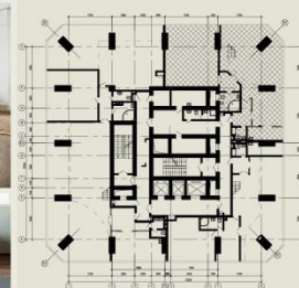
ПЛАН НА ОТМ. +101.400
