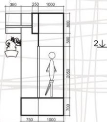
Разрез 1-1 М 1:25
