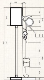
Разрез 1-1
