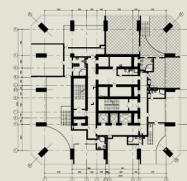
ПЛАН НА ОТМ. +98.700
