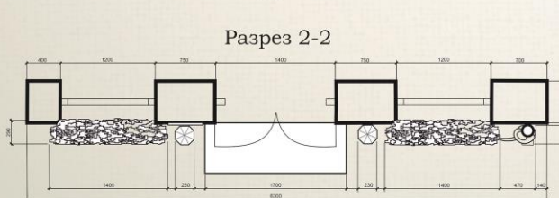
Разрез 2-2
