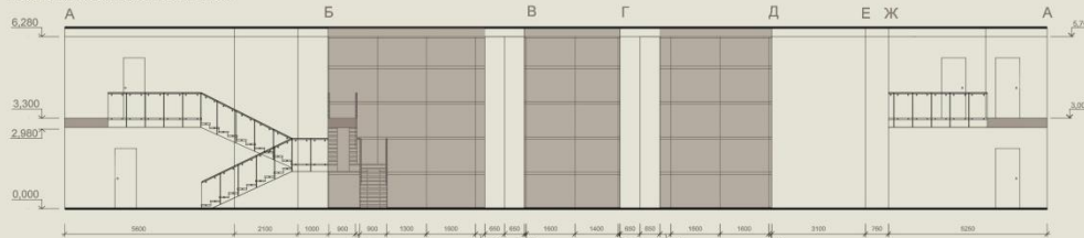
РАЗВЕРТКА СТЕН ГОСТИНОЙ М 1:50
