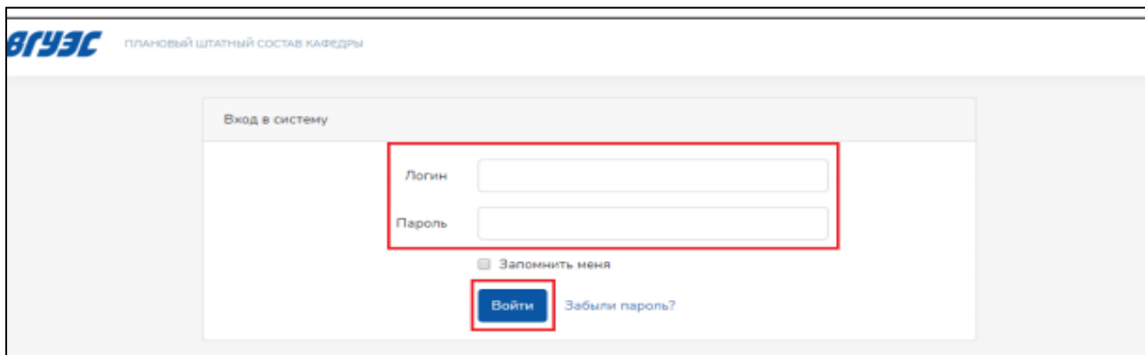
Рисунок 2 Авторизация
