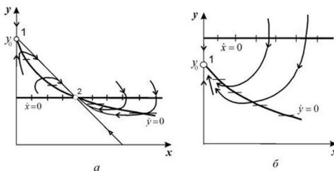
Рис. 11.4. Фазовые портреты системы 11.9. а – стационарный режим работы, б – режим вымывания.
