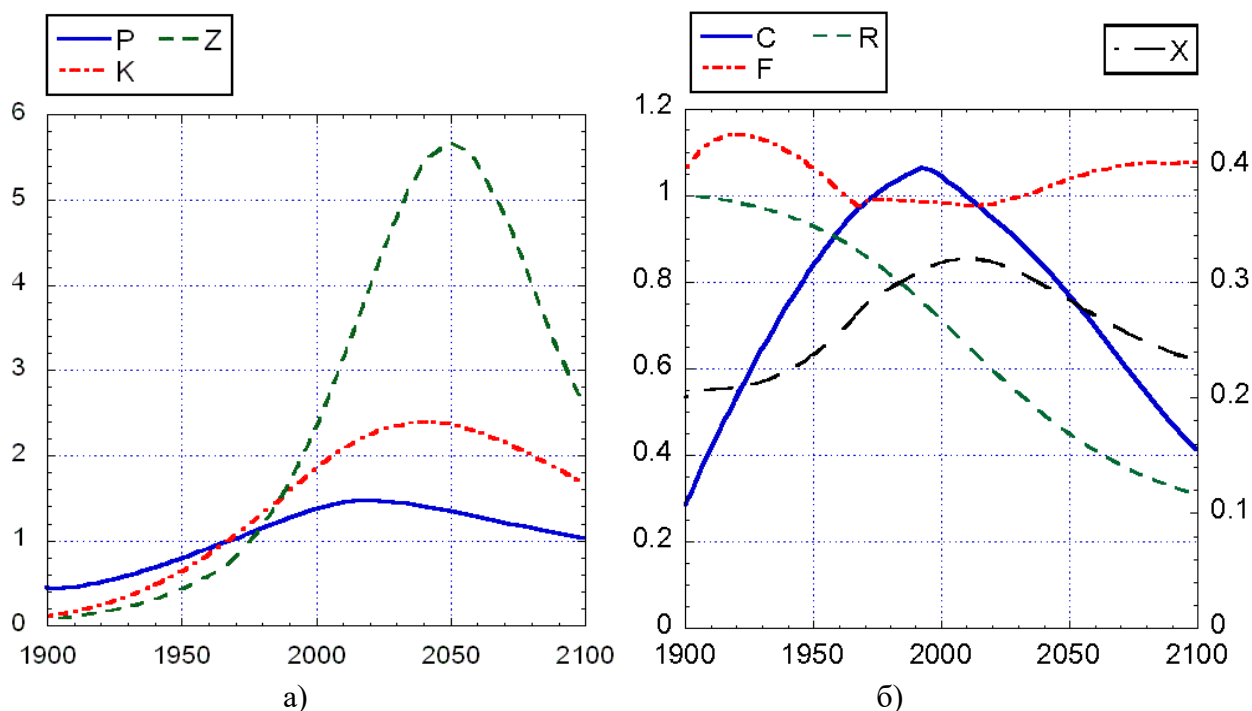
Рис. 3. Модель Форрестера в первоначальном виде: кризис ввиду истощения ресурсов. Сначала падает материальный уровень жизни, потом численность населения и капитал. Кризис наступает примерно к 2020-30 г.г. Все величины представлены в условных единицах (т.е. реально показаны не P, K, Z, R а P/P_N, K/P_N, Z/Z_N, R/R_0 соответственно). На рисунке б) графики представлены в двух масштабах: один показан на левой оси ординат, второй – на правой оси. Т.е., такие переменные, как уровень питания F , уровень жизни C и количество ресурсов R меняются от 0 до 1.2, а доля фондов в сельском хозяйстве – от 0 до 0.45.
